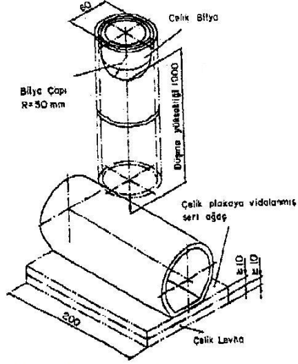
Şekil 6 Tünel Tipi Borularda Darbe Dayanımı Deneyi
